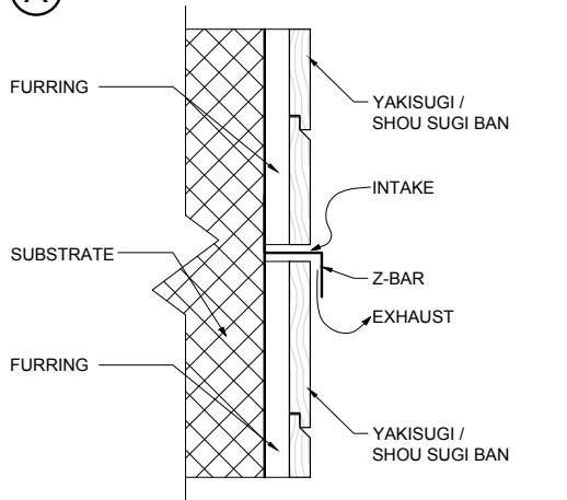
(D) HORIZONTAL LAYOUT BOND LINE VENTING
